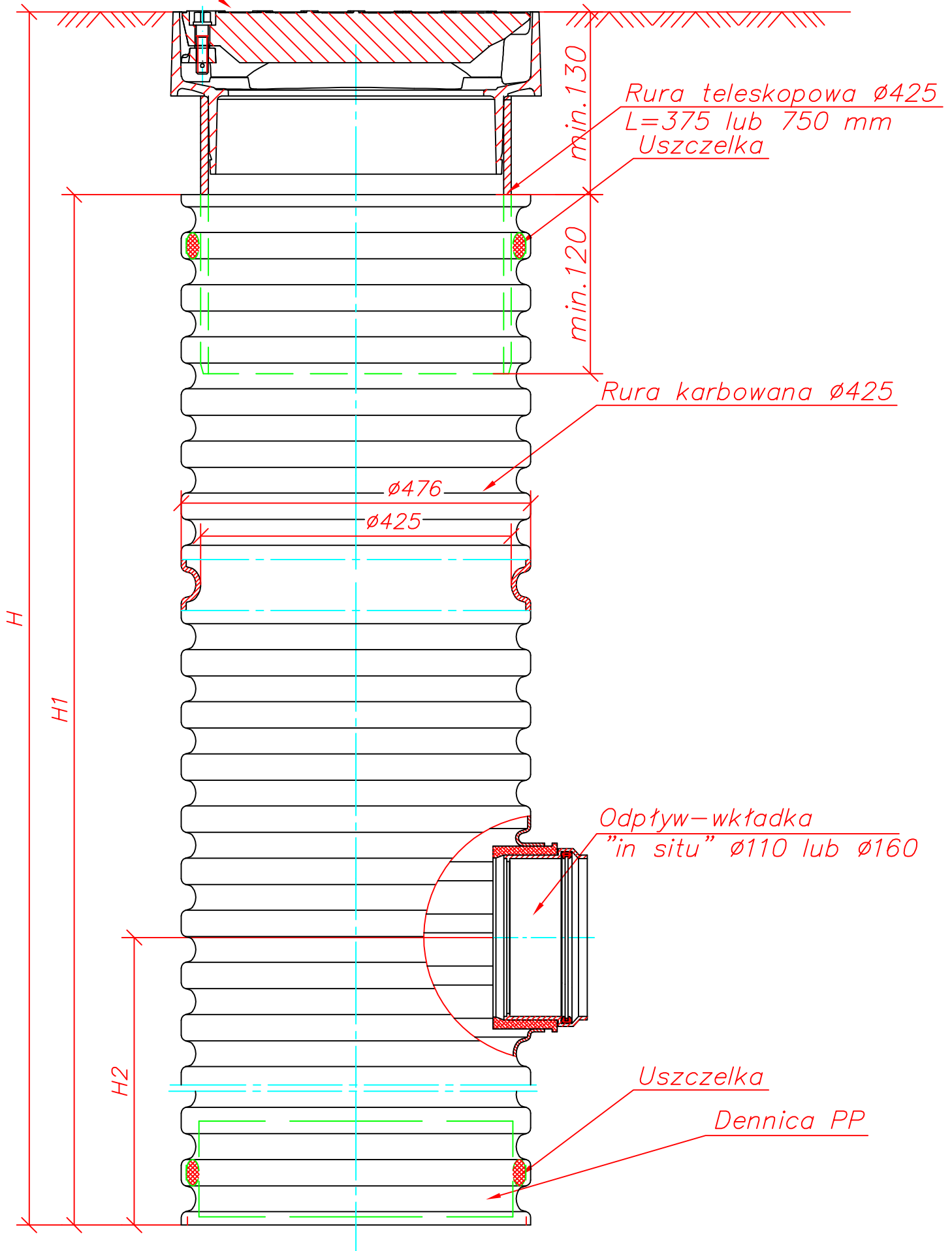
Studzienka osadnikowa \varnothing 425 ze wpustem klasy D400
